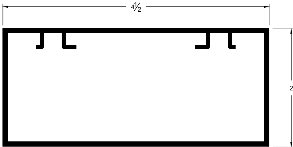
Header
