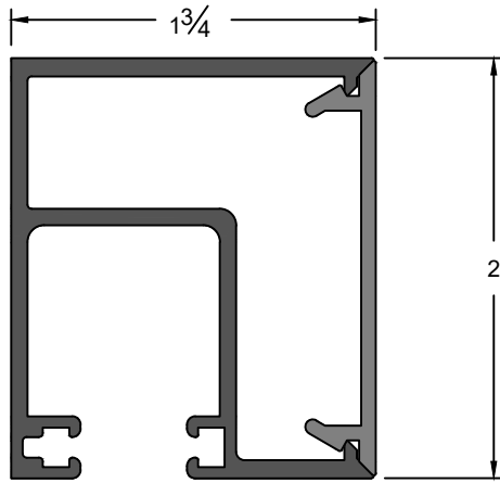
Wall Jamb Assembly
