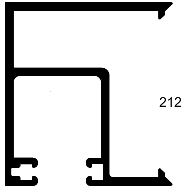
Wall Jamb
