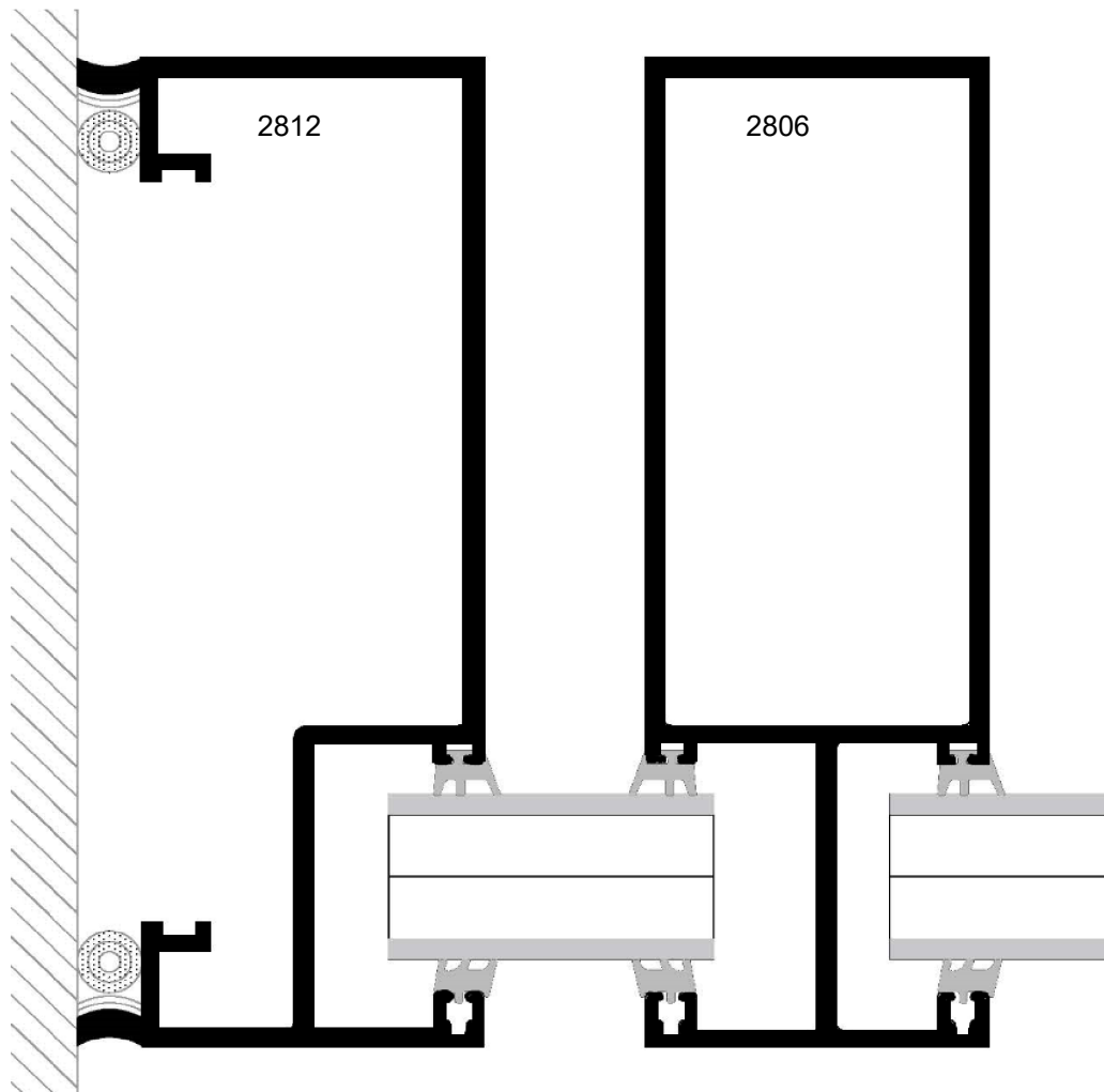
Wall Jamb
