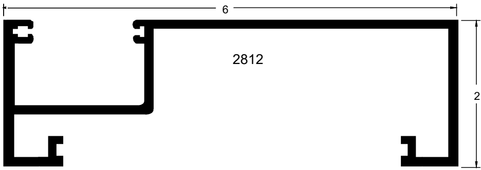
Wall Jamb
