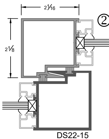
Interlock Stile
