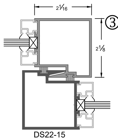
Interlock Stile
